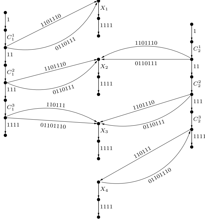
Fig. 9. Pattern \pi for the case when \phi = (x_1 \vee x_2 \vee \neg x_3) \wedge (x_2 \vee x_3 \vee \neg x_4) .
